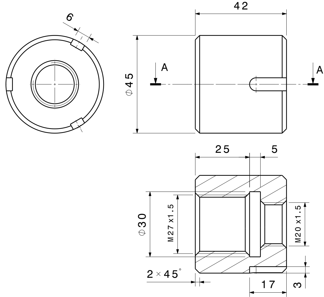
Vista A-A
